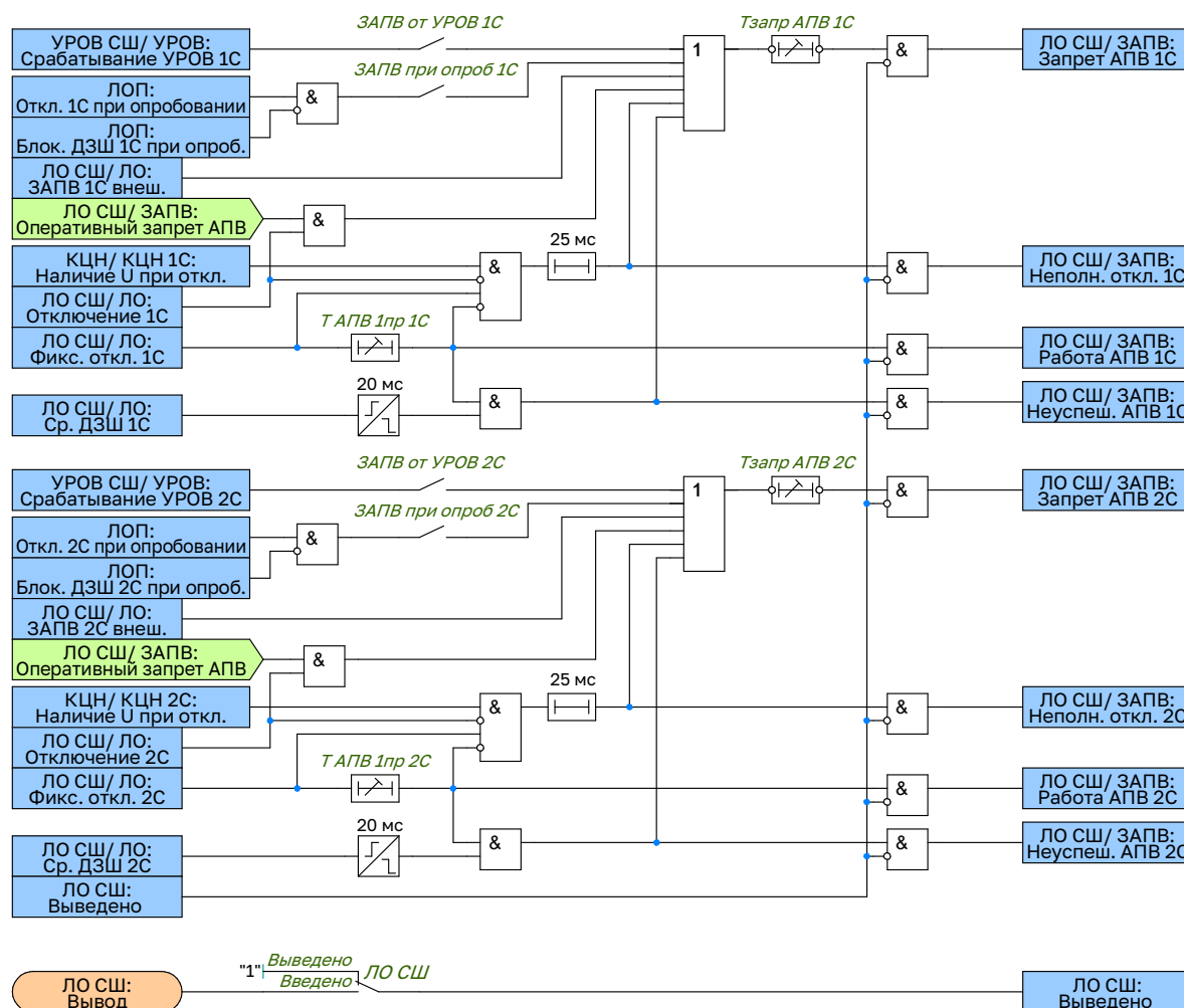
Рисунок 2.15 – Функциональная схема логики запрета АПВ
